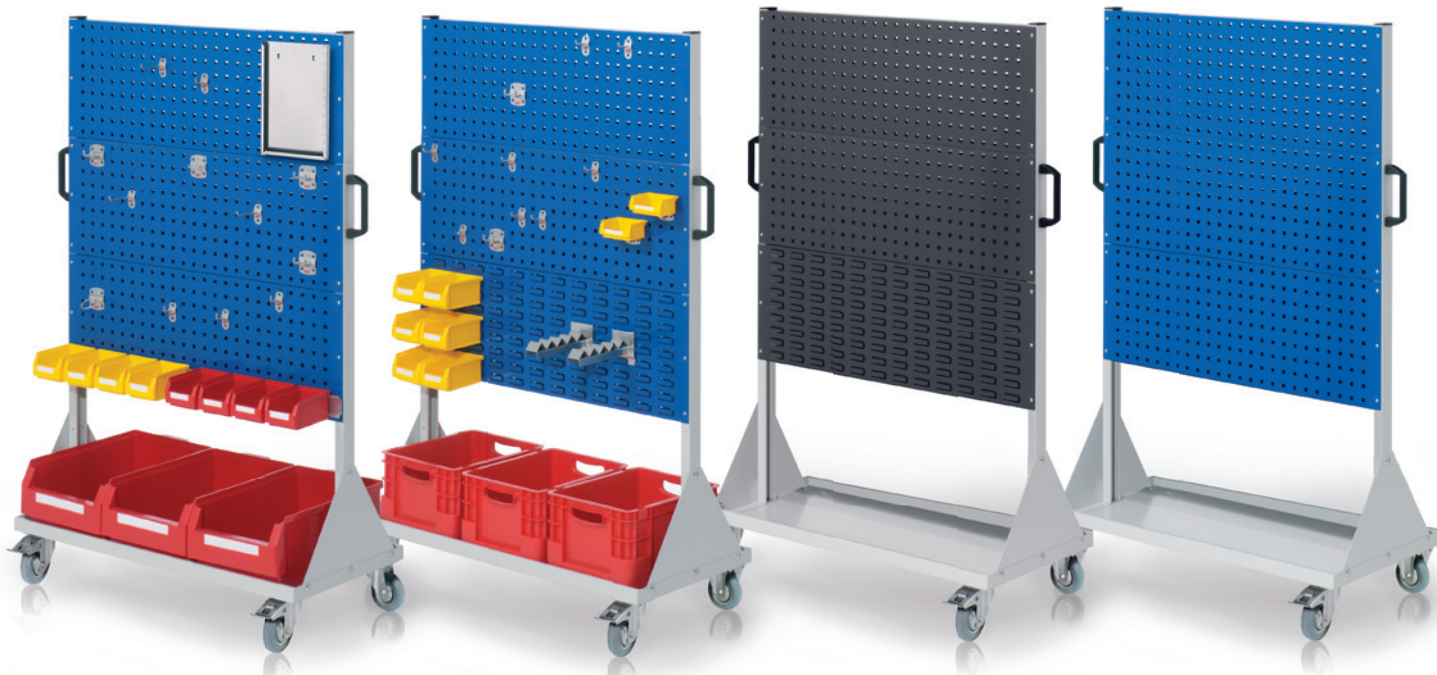
Chariots RasterMobil® Taille 4 - H 1580 x L 1000 x P 500 mm
